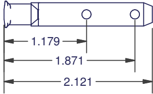
235 ZINC T-PIVOT
