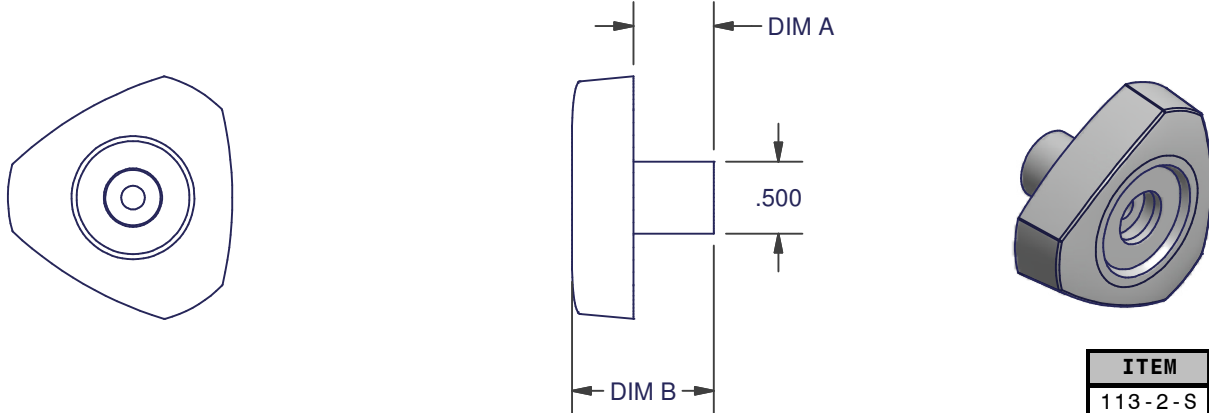
113-2 KNOB
